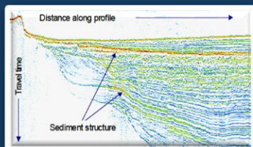
音波地層探査装置を用いた 海底の地層探査例
